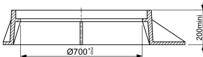
DOORSNEDE COUPE A-B
